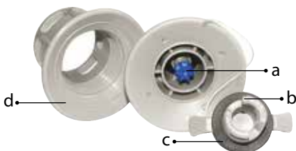
Фото воздушного клапана
